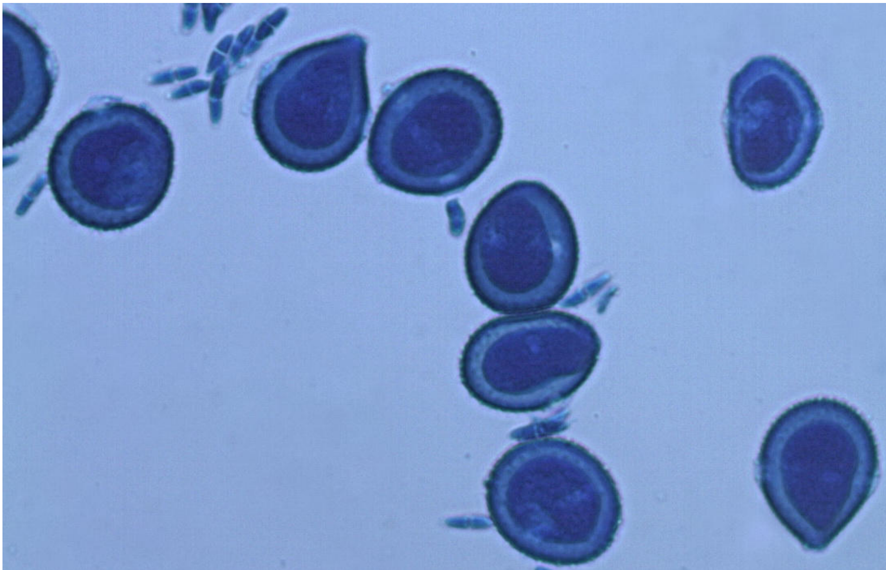
Urédospores : 27-34 x 24-28 \mu\text{m} , finement épineuses
